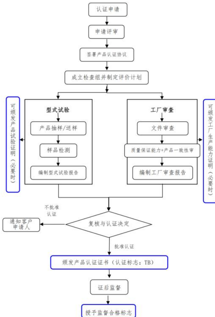
图 6-1 TB 型式认证工作流程图
